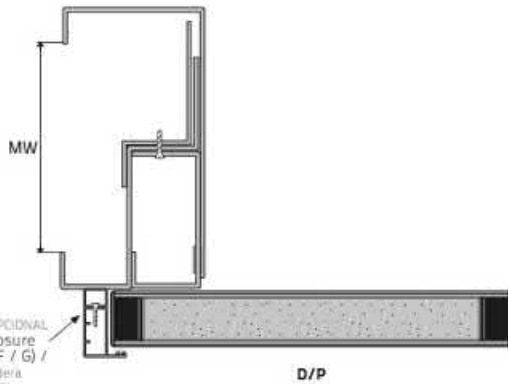
TYPE GH PROFILE PERFIL TIPO GH
