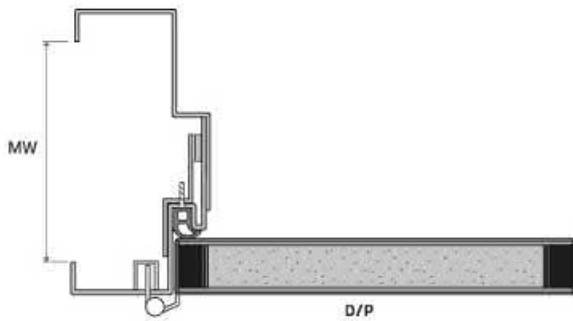
TYPE G7 PROFILE / PERFIL TIPO G7
