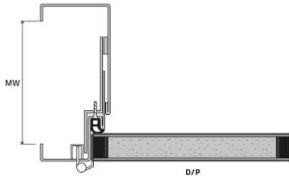
TYPE G7 PROFILE PERFIL TIPO G7
