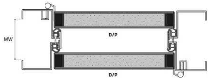
TYPE G-SHARED DOOR / TIPO G-COMUNICANTE
